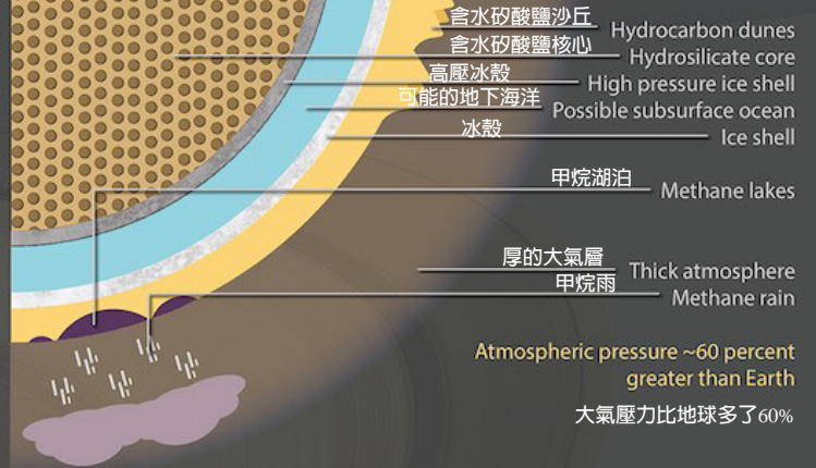
圖12. 地質活躍的衛星地質剖面圖。木衛一Io為多火山的環境、木衛二Europa冰殼下的大量鹹水海洋、土衛二Enceladus羽狀水蒸氣與高速冰粒噴流、土衛六Titan是擁有液態甲烷的星球。© NASA
